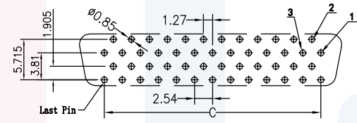
P.C. BOARD LAYOUT (50Pin) R1 Type / 正脚位
