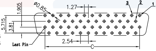
P.C. BOARD LAYOUT (50Pin) R2 Type / 反脚位
