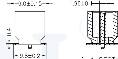
A-A SECTION
