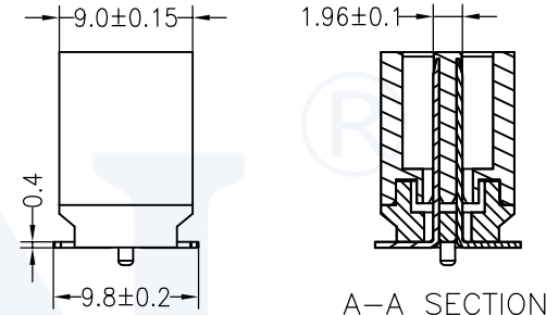
A-A SECTION
