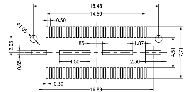
P.C.B Layout
