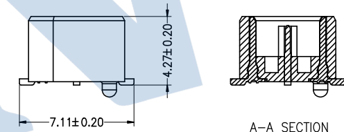
A-A SECTION
