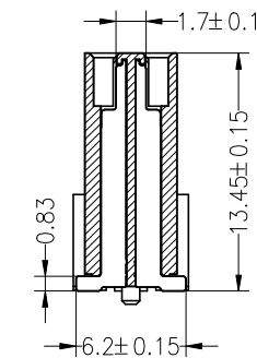
A-A SECTION
