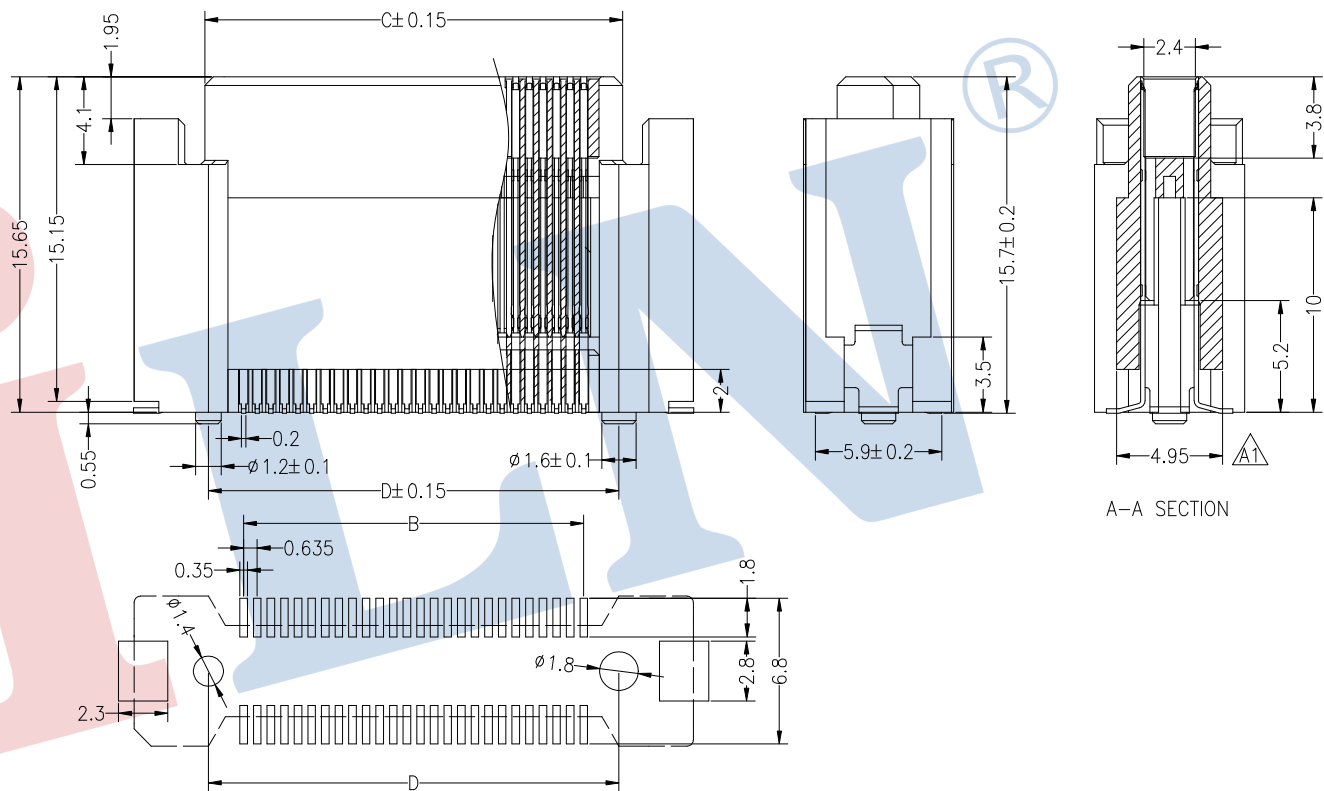
P.C.B Layout
