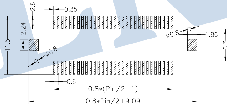
P.C.B Layout
